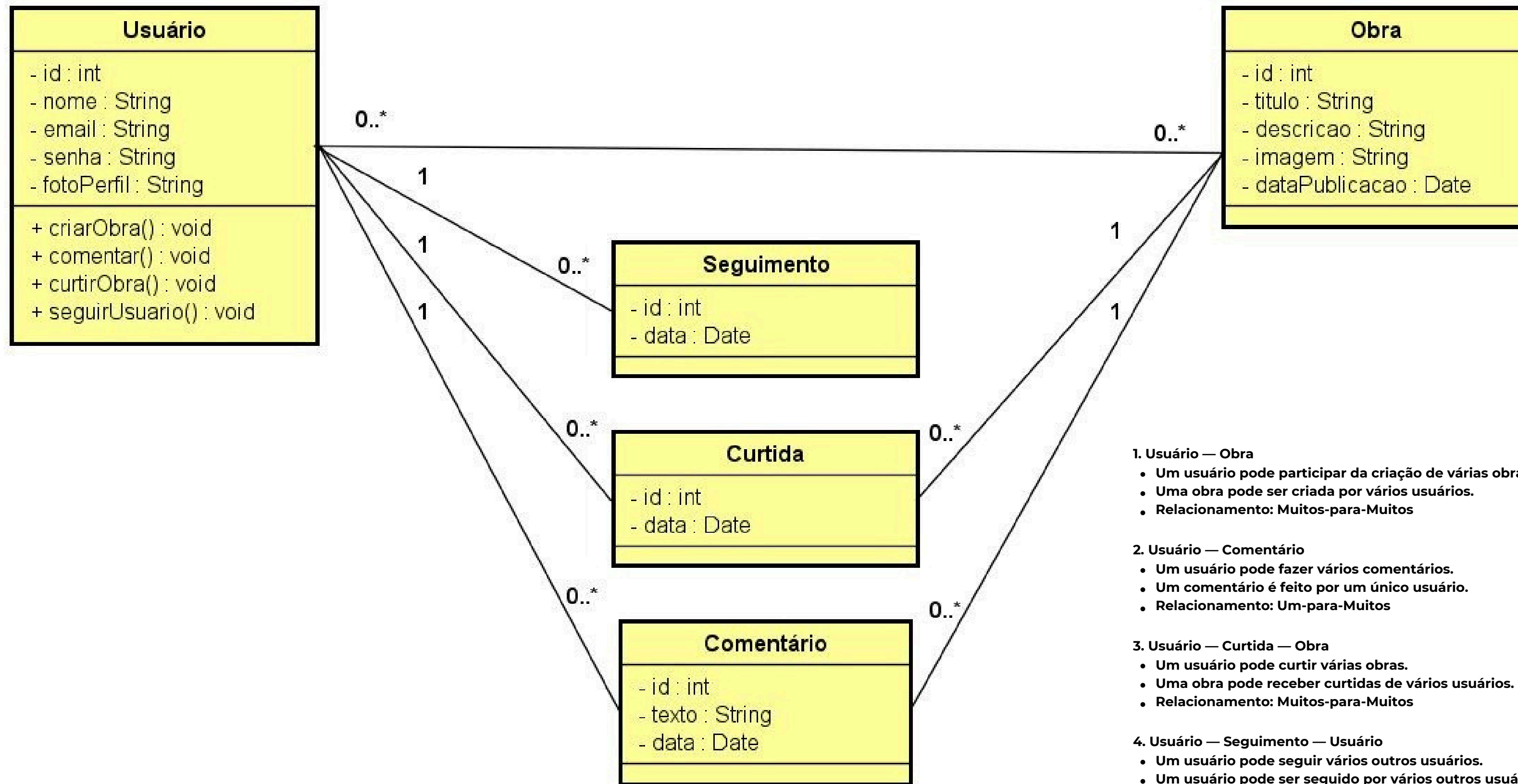
Diagrama de Classes
